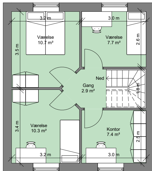
Boligplan type A 1. sal
