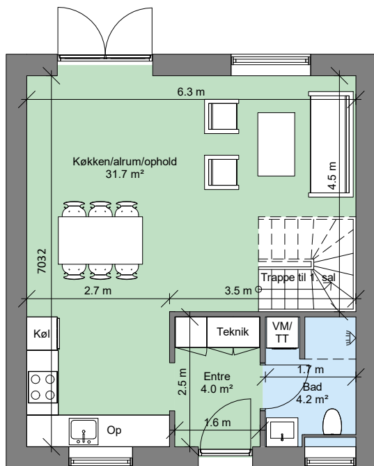
Boligplan type A stueplan
